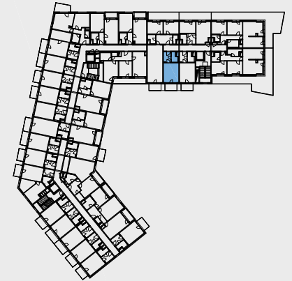
Půdorys podlaží, objekt A
