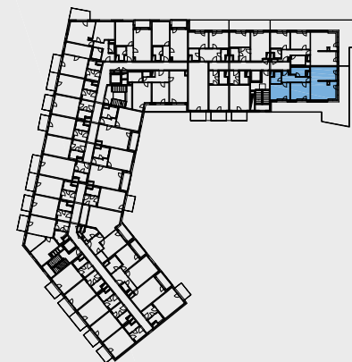
Půdorys podlaží, objekt A
