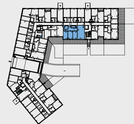
Půdorys podlaží, objekt A
