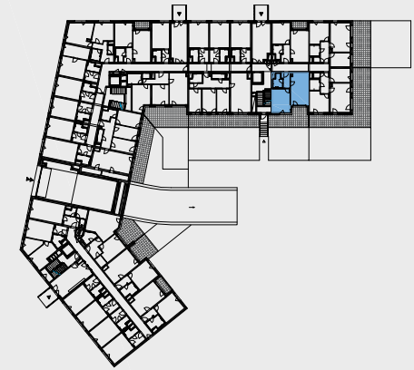
Půdorys podlaží, objekt A
